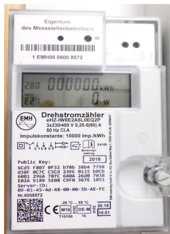
Stromzähler
