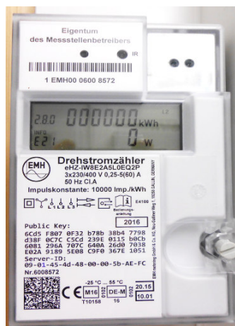
Stromzähler
