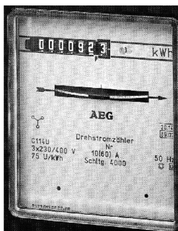
Stromzähler
